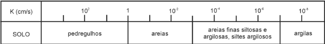
Figura 2 – Estimativa da permeabilidade dos solos com base na granulometria do material. Fonte: de acordo com a fórmula de Hazen (apud MELLO, TEIXEIRA, 1967)).
