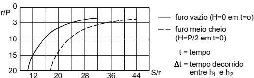
Figura 15 – Ensaios de rebaixamento e recuperação em sondagens.
