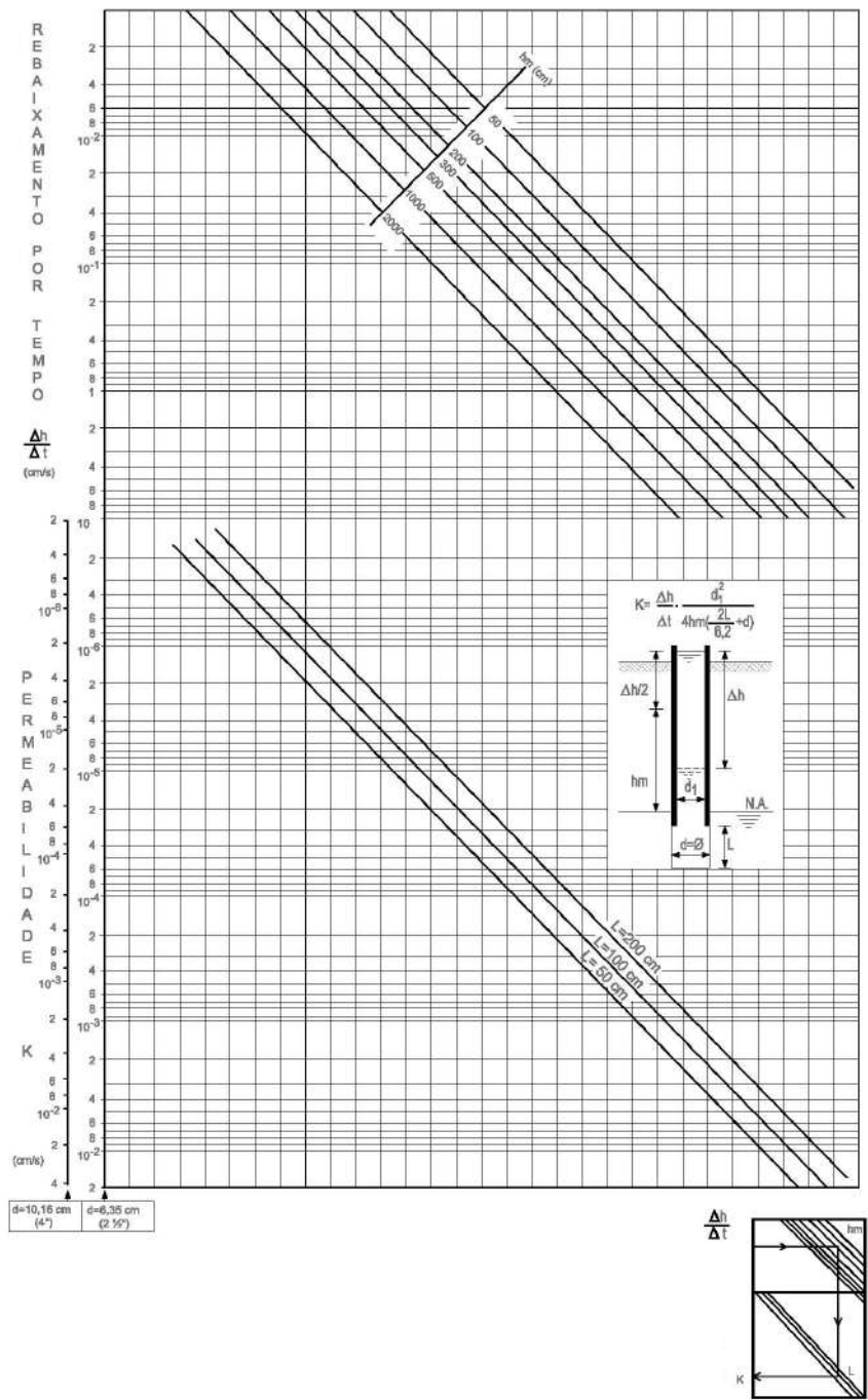
Figura 21 – Ábaco para cálculo de ensaios de rebaixamento para trechos de ensaios situados acima do N.A.
