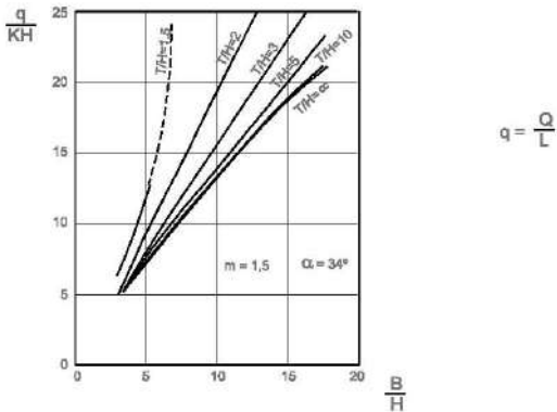
Figura 22 – Ensaios de cava – parâmetros e variáveis utilizadas na determinação de permeabilidade.
