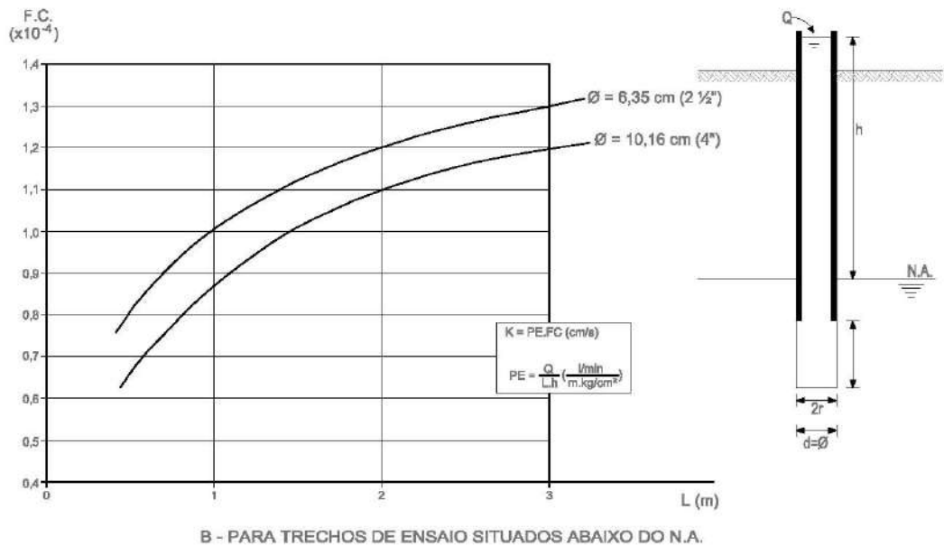
Figura 19 – Ensaios de infiltração. Ábacos para conversão de perda d’água específica (PE) em permeabilidade (K).
