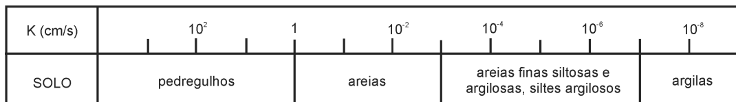
Figura 2 – Estimativa da permeabilidade dos solos com base na granulometria do material.
