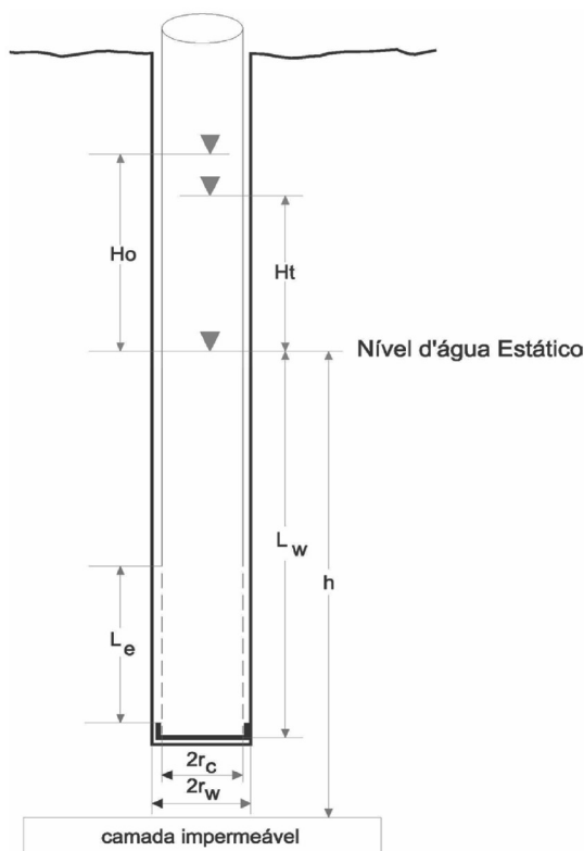
Figura 10 – Geometria e notações de um poço parcialmente penetrante em um aquífero livre, após a elevação do nível d'água.
